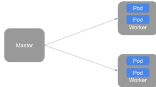
圖4. Kubernetes 架構
